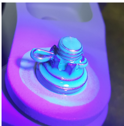
CPC ARDROX AV 40 INSPECTION WITH A UV LIGHT
